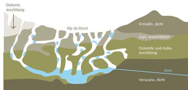
Geologische Situation des Karstgebietes bei Alp da Munt
